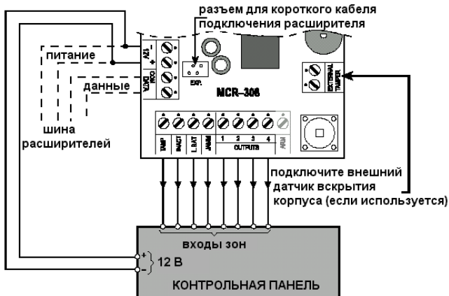
Рисунок 5. Схема подключения
