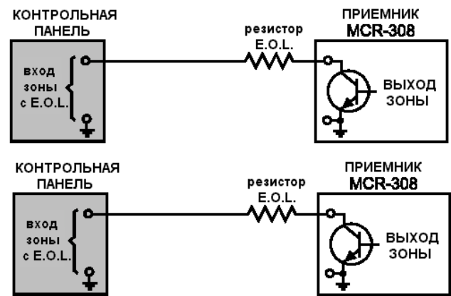
Рисунок 6. Подключение к панели, имеющей оконечные сопротивления
