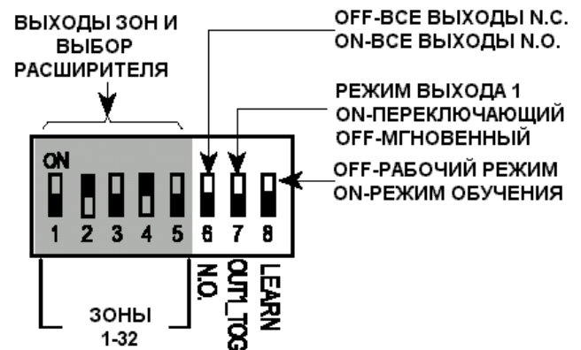
Рисунок 7. Назначение DIP-переключателей
